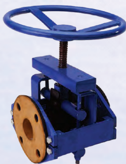
Válvula Pinch
